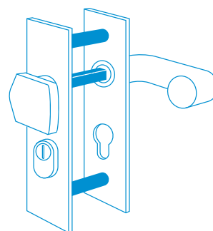
De harde metalen bescherming van het veiligheidsbeslag met cilindertrekbeveiliging is duidelijk herkenbaar en schrikt inbrekers af.
